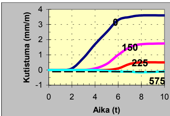
Kuva 4. Betonipinnan plastinen kutistuma erisuuruuksilla varhaisjälkihoitoaineen ruiskutusmäärillä, tuulen nopeus 2,5 m/s, T=20 °C, 40 % RH /1/.
